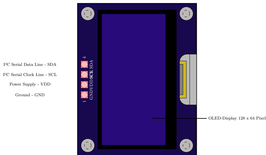
Abbildung 7.1.: OLED-Display nach fig:OLEDsketch
